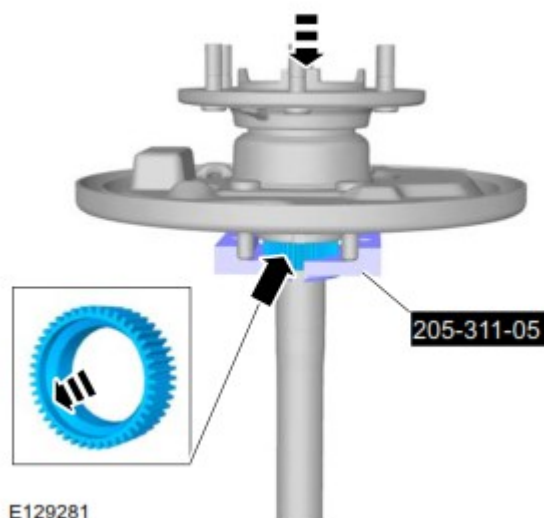
Abbildung 4: Blau ABS Ring HA
