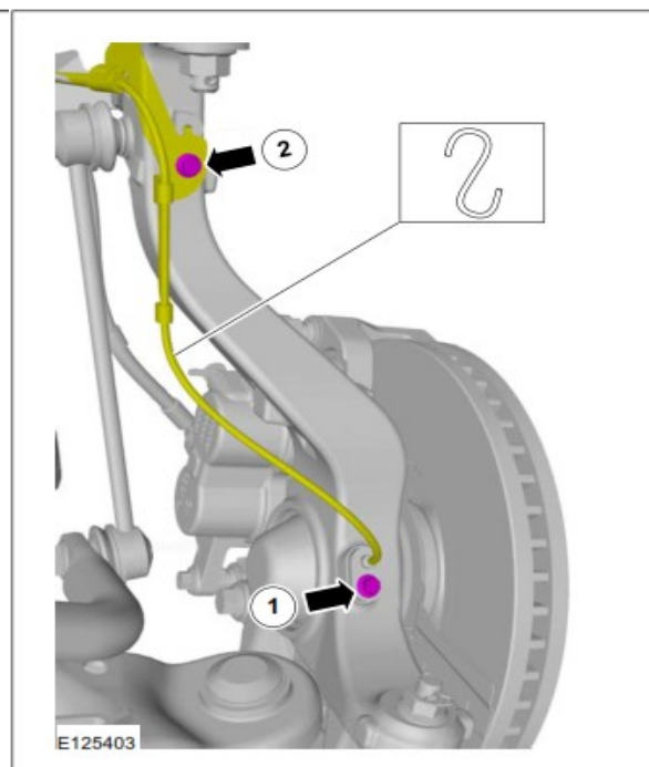
Abbildung 2: 1 ABS Sensor 2 Befestigung Kabel
