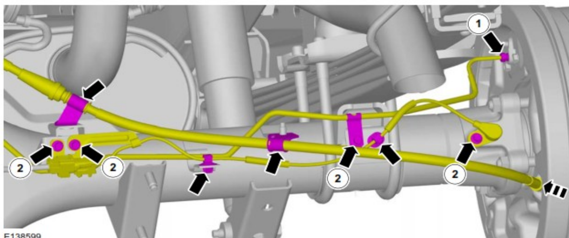
Abbildung 3: 2 ABS Sensor Hinterachse
