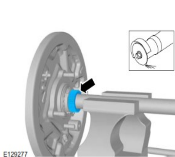
Abbildung 5: Blau ABS-Ring HA
