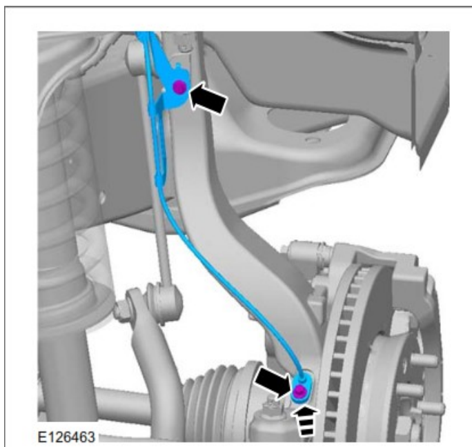
Abbildung 1: ABS Sensor und Kabel Vorderachse
